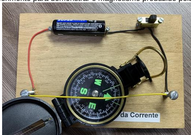
Imagem 3 – Experimento para demonstrar o magnetismo produzido pela corrente elétrica.
