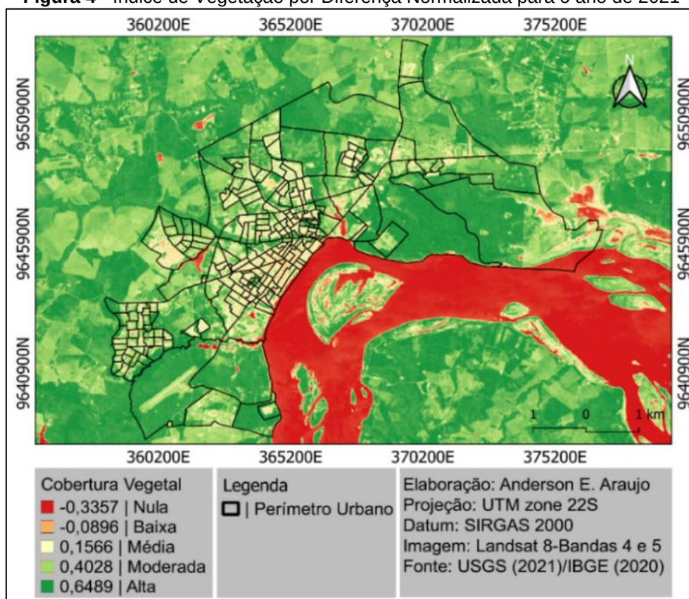
Figura 4 - Índice de Vegetação por Diferença Normalizada para o ano de 2021
