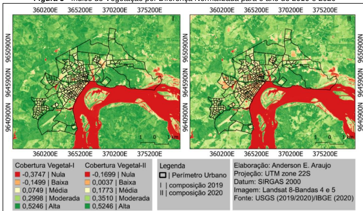
Figura 3 - Índice de Vegetação por Diferença Normalizada para o ano de 2019 e 2020
