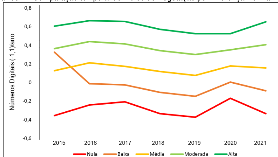
Gráfico 1 - Comparação temporal do Índice de Vegetação por Diferença Normalizada.
